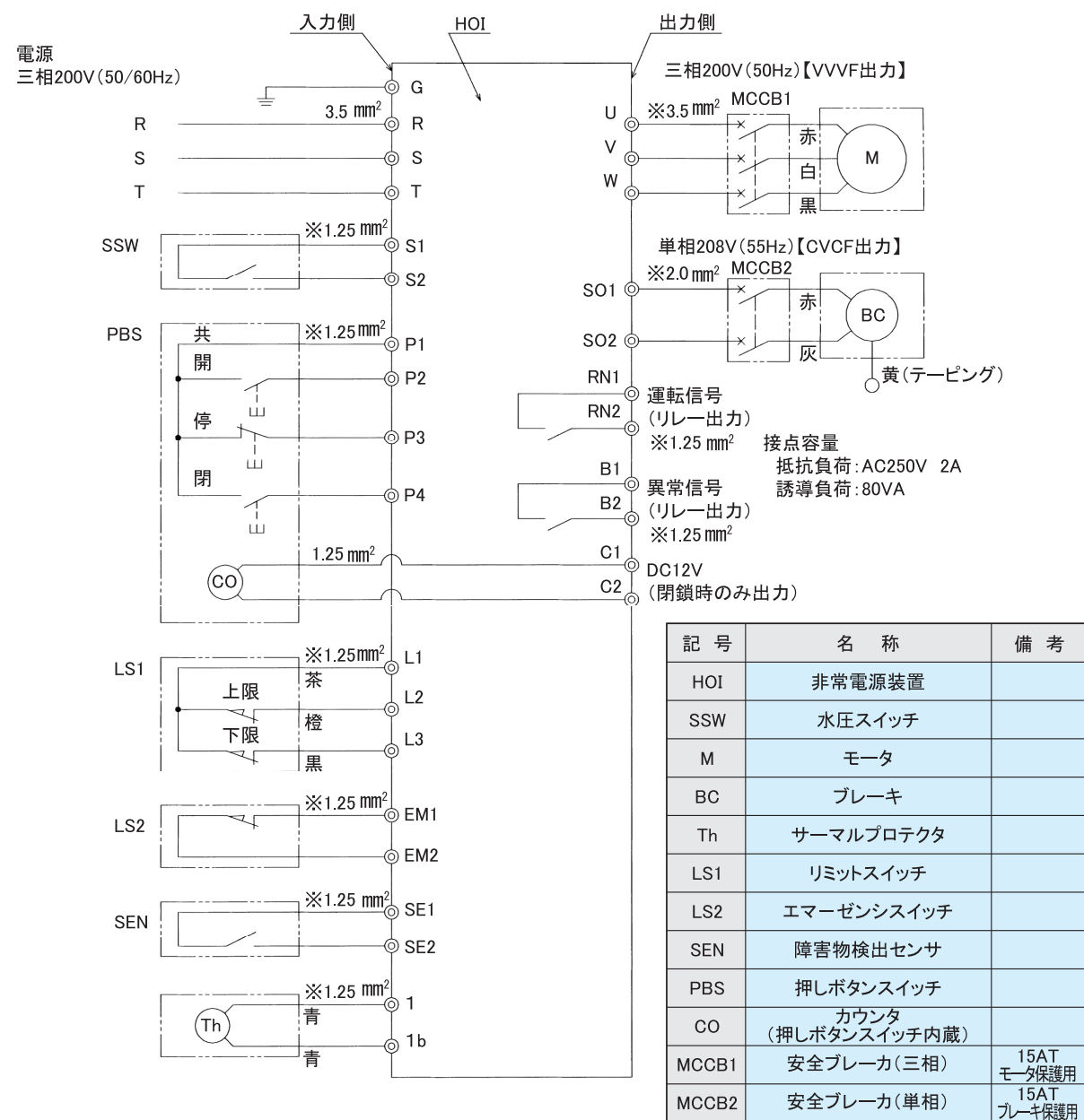
【結線図】
