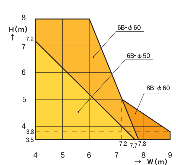
○スラット板厚1.4mm（ピッチ100mm）の場合 1.4mm thick slat (pitch 100mm) in use
