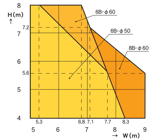
○スラット板厚1.6mm（ピッチ75mm）の場合 1.6mm thick slat (pitch 75mm) in use
