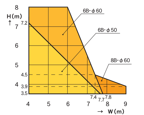
○スラット板厚1.4mm（ピッチ100mm）の場合 1.4mm thick slat (pitch 100mm) in use
