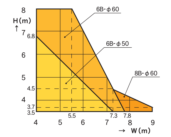
○スラット板厚1.6mm（ピッチ100mm）の場合 1.6mm thick slat (pitch 100mm) in use
