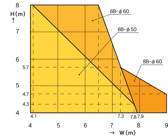
○防煙スラット板厚1.6mmの場合 1.6mm thick smoke-proof slat in use
