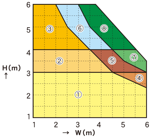
○スラット 板厚1.2mm(ピッチ75mm)の場合 1.2mm thick slat (pitch 75mm) in use
