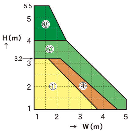
○スラット 板厚1.5mm(ピッチ75mm)の場合 1.5mm thick slat (pitch 75mm) in use
