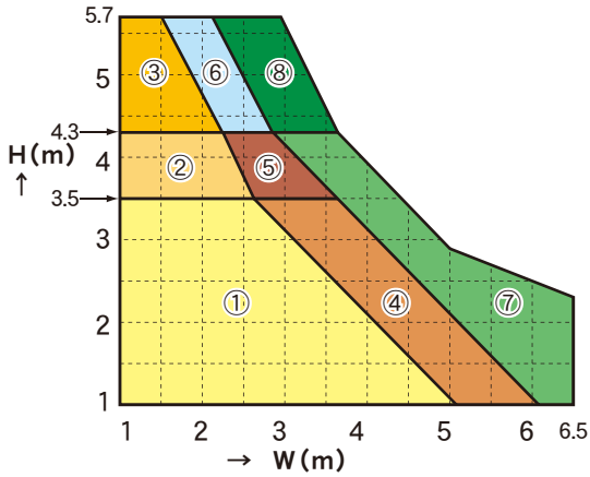
○スラット 板厚1.0mm(ピッチ75mm)の場合 1.0mm thick slat (pitch 75mm) in use
