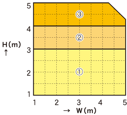
○スラット 板厚1.0mm(ピッチ75mm)の場合 1.0mm thick slat (pitch 75mm) in use
