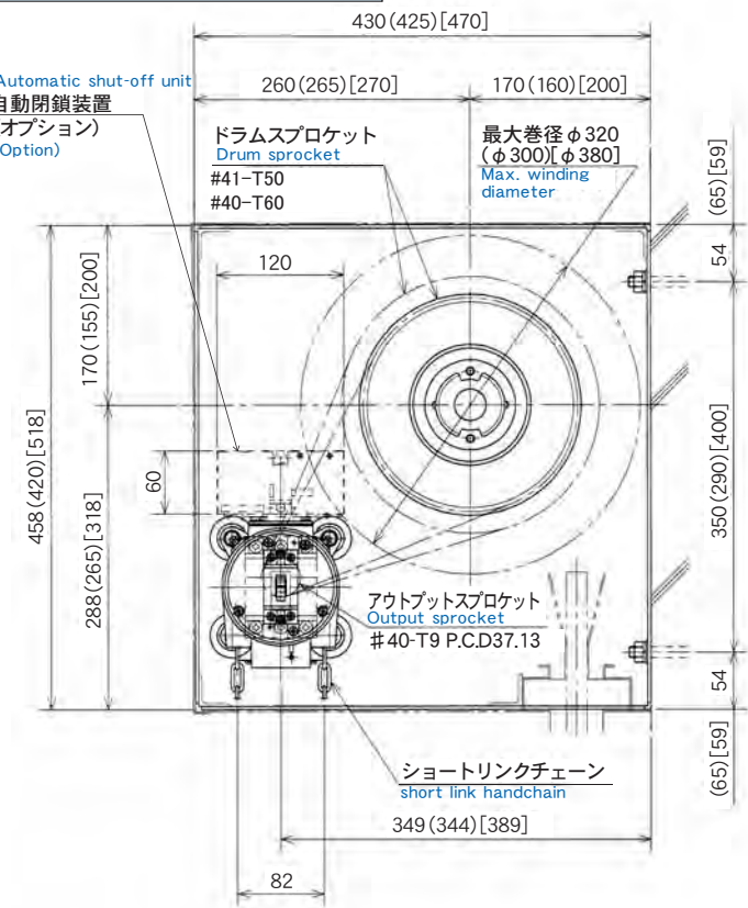
BK型ブラケット BK type bracket
