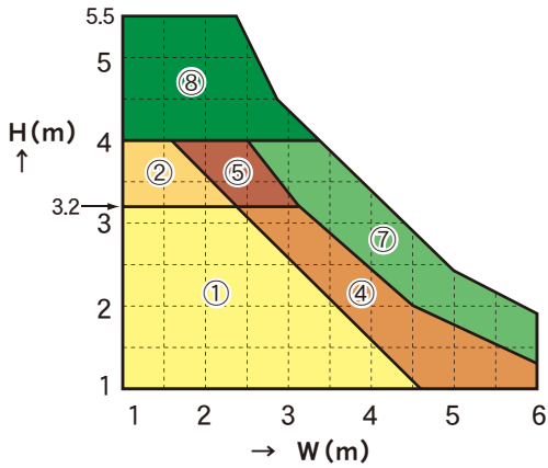
○スラット 板厚1.5mm(ピッチ75mm)の場合 1.5mm thick slat (pitch 75mm) in use
