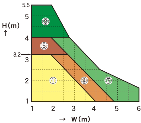
○スラット 板厚1.4mm(ピッチ75mm)の場合 1.4mm thick slat (pitch 75mm) in use
