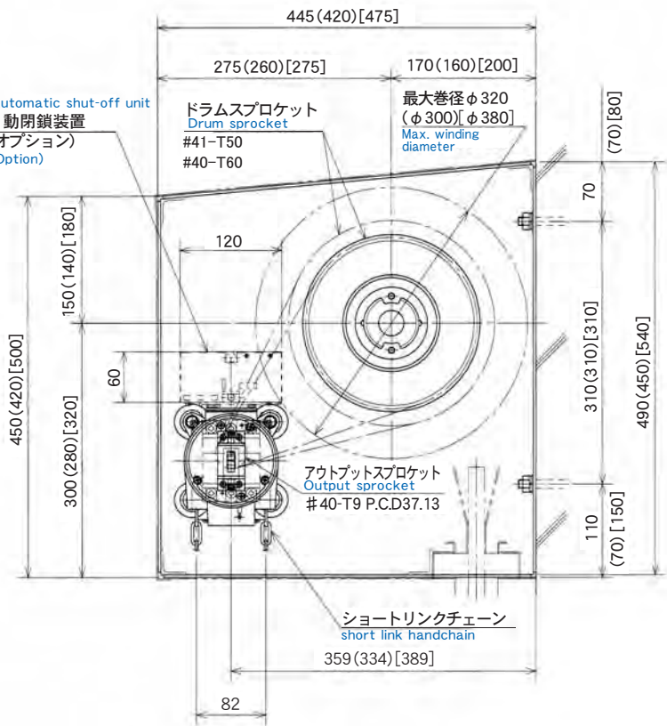
BC型ブラケット BC type bracket
