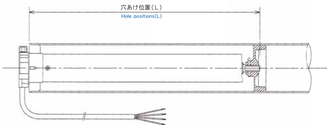
L寸法 Dimension L
