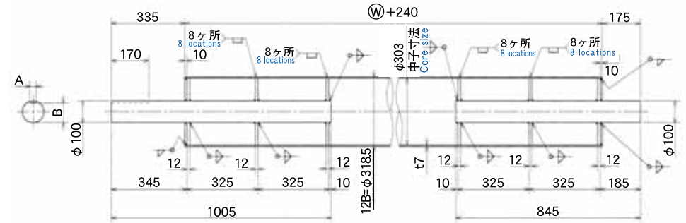
【12B 巻取ドラム寸法】 【12B Winding drum dimension】
