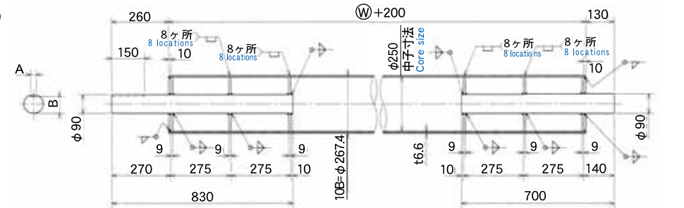
【10B 巻取ドラム寸法】 【10B Winding drum dimension】
