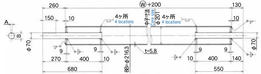
【8B 巻取ドラム寸法】 【8B Winding drum dimension】
