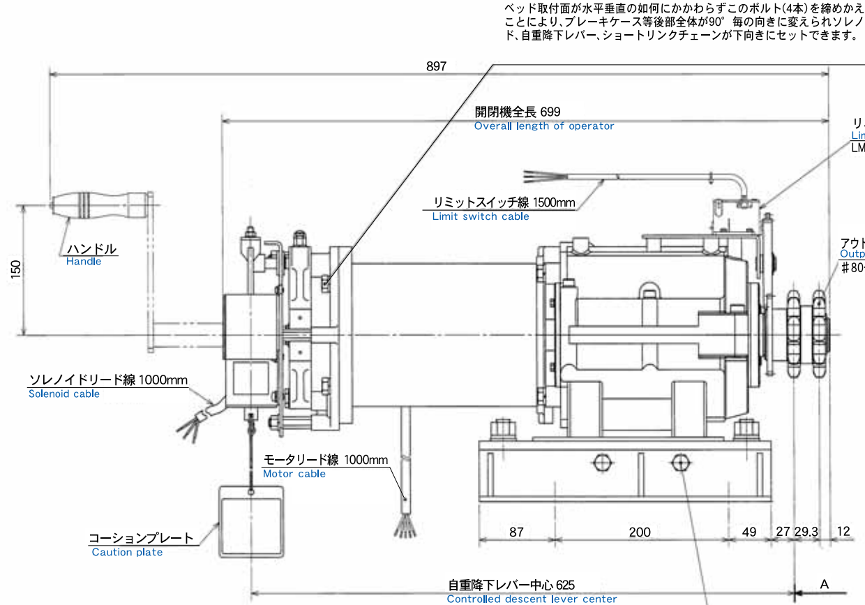
ハンドル式 Handcrank manual type
