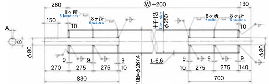
【10B 巻取ドラム寸法】 【10B Winding drum dimension】
